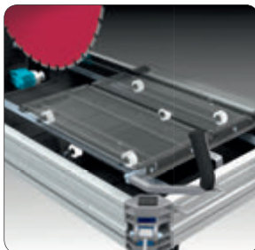
Zaagwagen met 6 gelagerde wielen
